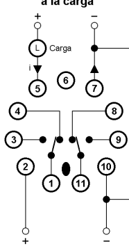
Alimentación CC
