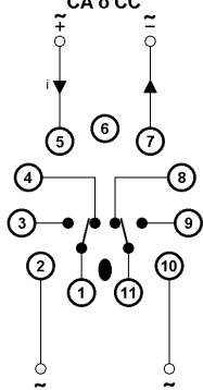
Alimentación CA
